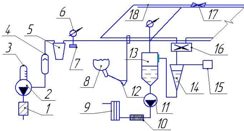
Доильная установка с молокопроводом
