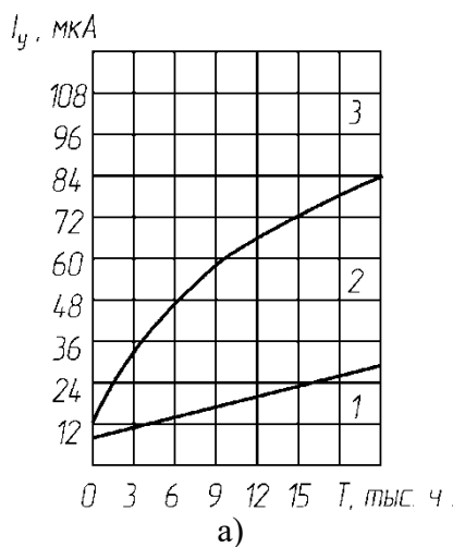
Рисунок - Области значений токов утечки (а) и тангенса угла диэлектрических потерь (б) для трех групп технического состояния изоляции погружных электродвигателей:
