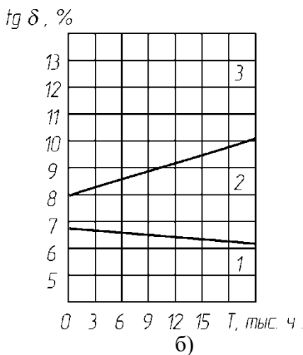
Рисунок - Области значений токов утечки (а) и тангенса угла диэлектрических потерь (б) для трех групп технического состояния изоляции погружных электродвигателей:
