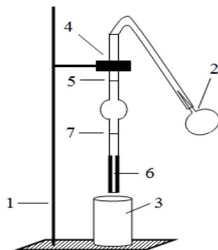
Рисунок 1. Установка для определения поверхностного натяжения.
