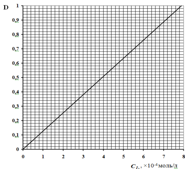
Рисунок 1. Градуировочный график для определения концентрации иода.
